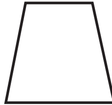
trapezium
